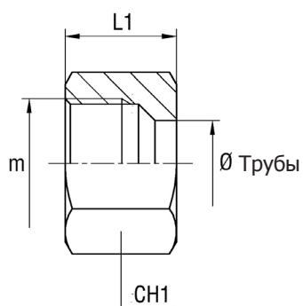
Гайка обжимная Арт.1002
