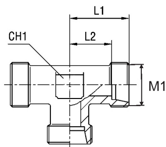
Фитинг тройник Арт. 1039..1
