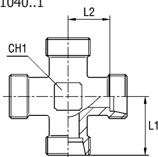
Фитинг четверник Арт. 1040..1
