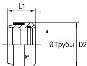
Кольцо врезное "В4" Арт.1001..4
