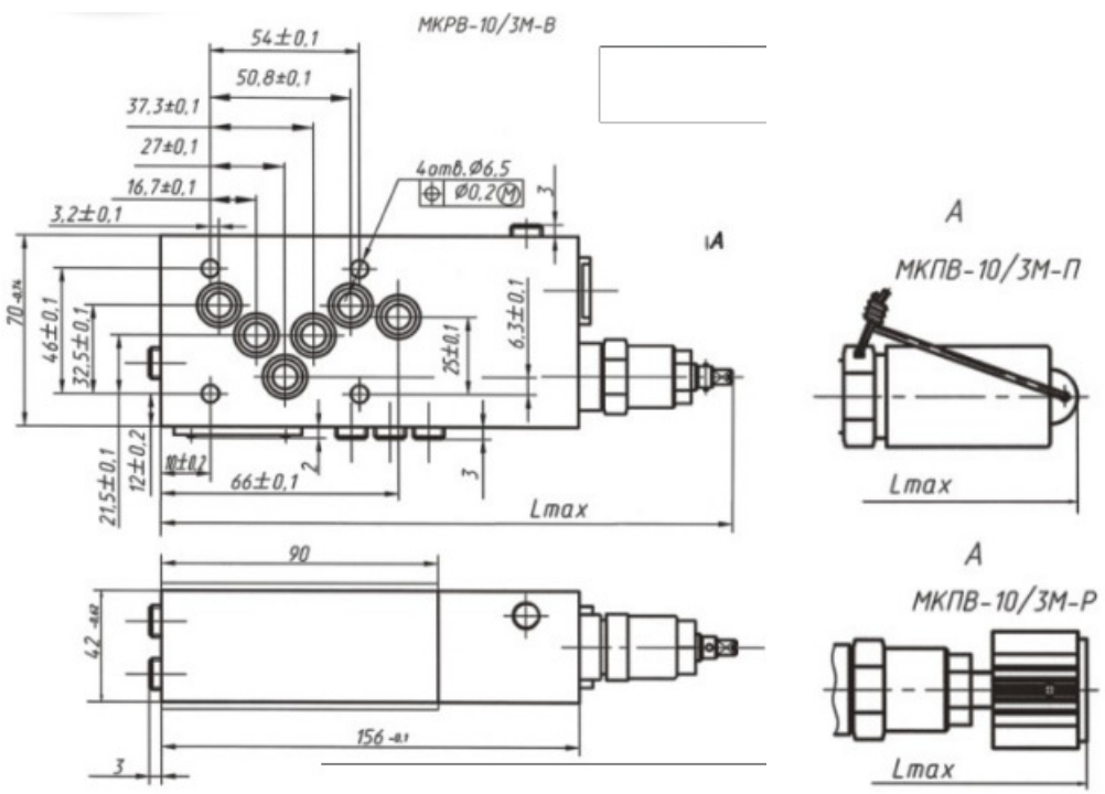
Общий вид, габаритные и присоединительные размеры гидроклапанов редукционных МКРВ-10/3М
